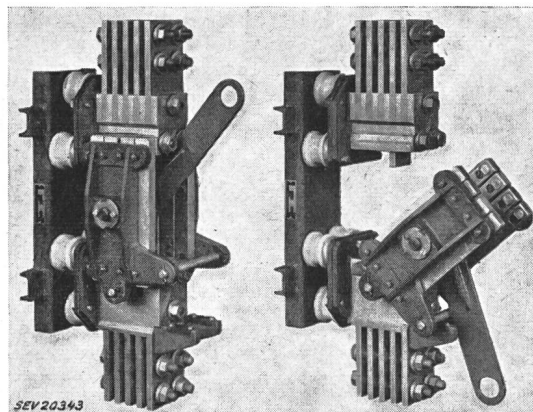
Fig. 2 Trenner für grosse Stromstärken
