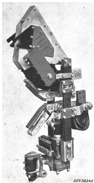
Fig. 4 Hüpf für Stromstärken bis 2500 A
