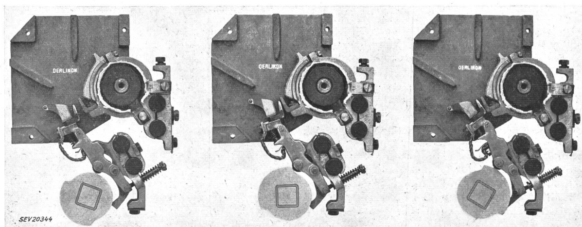
Fig. 3 Element eines Strassenbahn-Fahrschalters in 3 verschiedenen Stellungen
