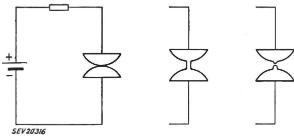
Fig. 5 Funkenfreie Kontakttrennung Feinwanderung
