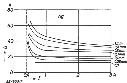
Fig. 4 Lichtbogencharakteristik für eingelaufene Silberkontakte mit dem Kontaktabstand als Parameter (nach Holm)
