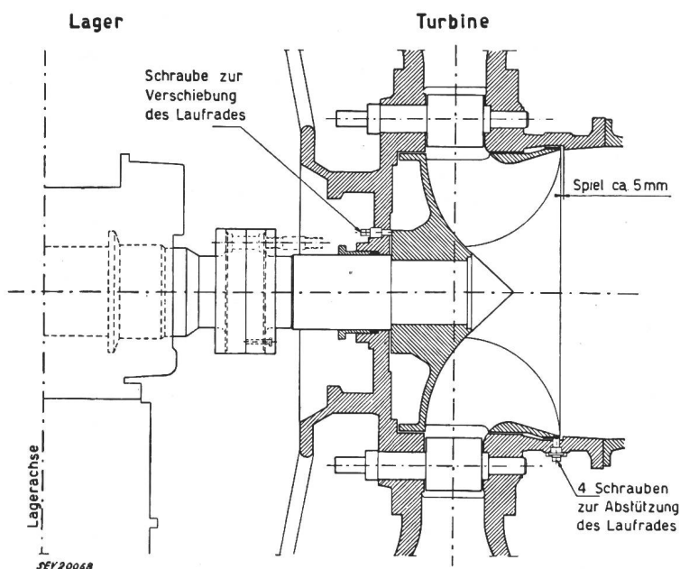
Fig. 15 Turbine, schematischer Schnitt mit Verschlebe- und Stützschauben
