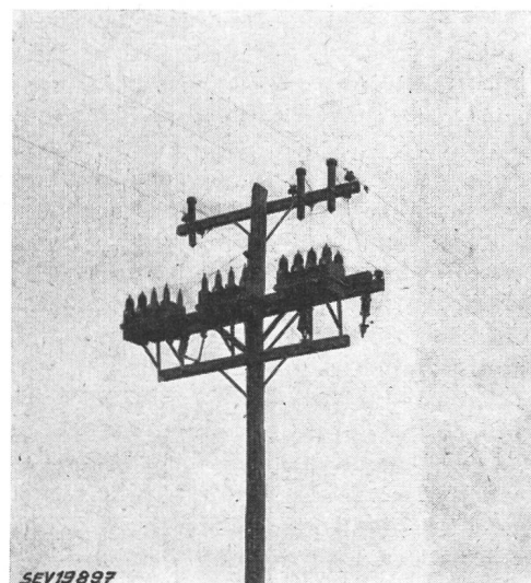
Fig. 7 180-kVar-Kondensatorenbatterie
