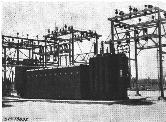
Fig. 2 Einheits-Unterwerk mit zwei 3025-kVA-Transformatoren, 33/2,4 kV Im Hintergrund links sind die Ölschalter sichtbar
