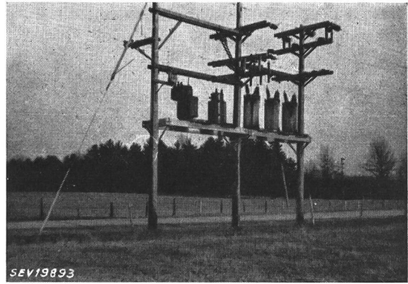
Fig. 3 Einfache Transformatorstation bestehend aus drei 100-kVA-Transformatoren, 33/2,4 kV Daneben ein 50-kVA-Transformator, 2,4 kV, 120/240 V. Links aussen ist ein Spannungsregulator sichtbar
