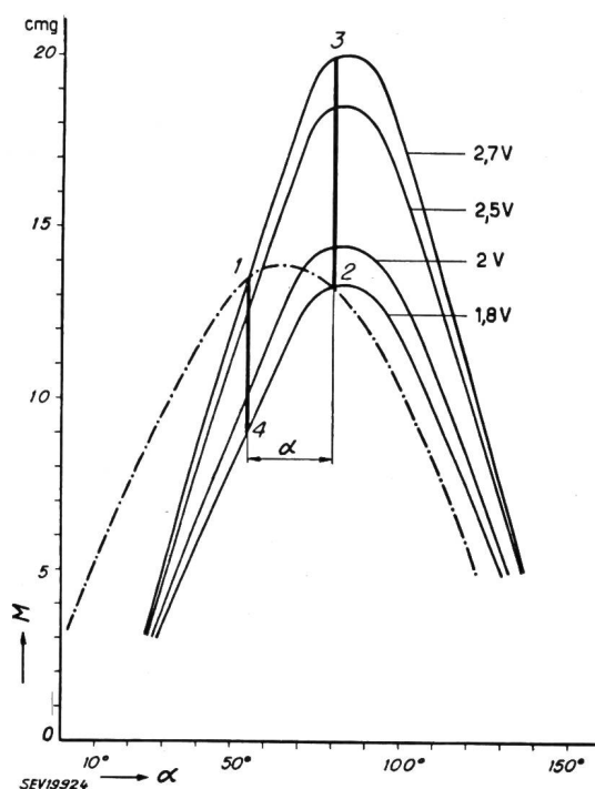
Fig. 2 Drehmomente M des Feder- und des beweglichen Systems als Funktion des Verdrehungswinkels \alpha - - - - - Drehmoment der Federkraft ———— Drehmomente des Systems \alpha Verdrehungswinkel
