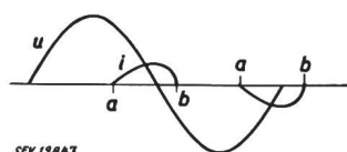
Fig. 1 Allgemeinster Fall der Arbeitsweise eines elektrischen Ventils Erklärungen siehe im Text
