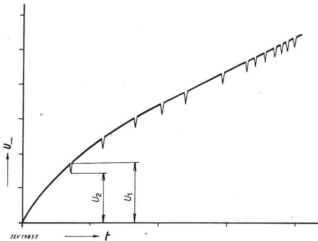
Fig. 3 Spannungsverlauf beim Durchschlagen von Metallpapier in Abhängigkeit der Spannungshöhe U Spannung; t Zeit
