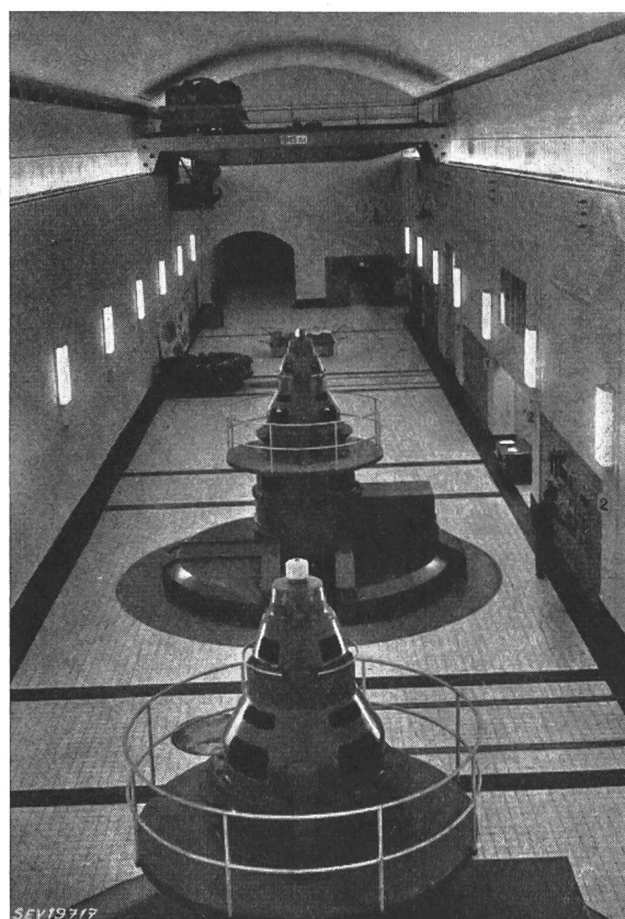
Fig. 7 Maschinenaal Handeck II Ansicht aus Kranbahnhöhe
