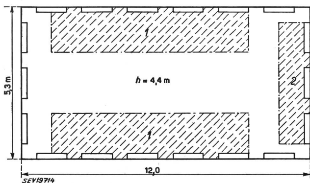
Fig. 4 Werkstatt Handeck II (Grundriss) Allgemeine Beleuchtung 18 Lampen FL 40 1 Werkzeugmaschinen; 2 Werkbank
