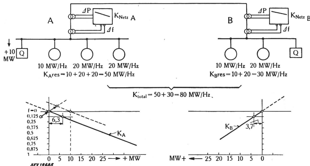
Fig. 3 Prinzipschema der Regulierung mittels Netz-Kennlinien-Regler
