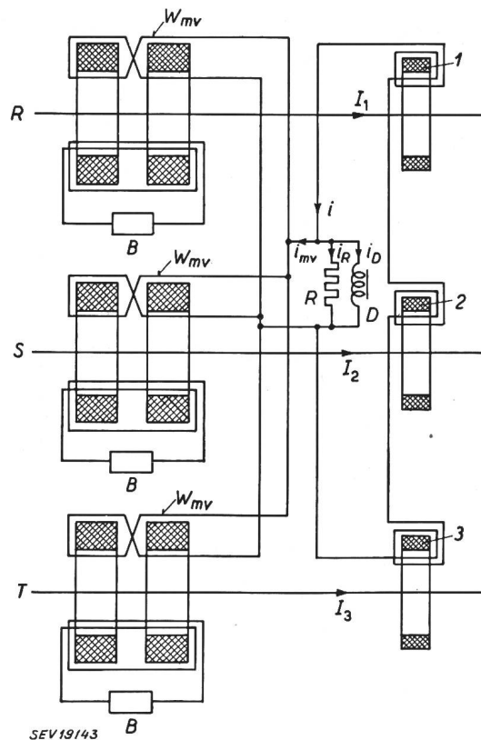
Fig. 3 Schaltung nach Vorschlag des Verfassers W_{mv} Vormagnetisierungswicklungen; B Bürden; R Ohmscher Widerstand; D Drosselspule; 1, 2, 3 Hilfskerne
