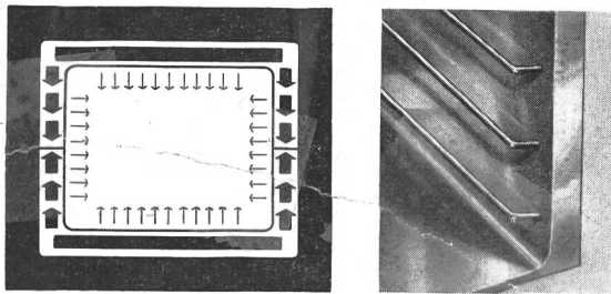
Fig. 4 Neuer Backofen links: Wärmeverteilung rechts: Ausschnitt
