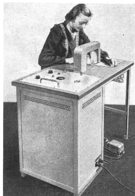
Fig. 1 Plastic-Näh-Schweissmaschine (HF-Generator für dielektrische Heizung)
