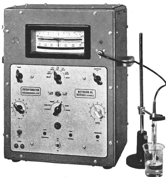
Fig. 2 Präzisionspotentiometer
