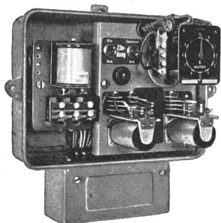
Fig. 2 Ölfeuerungsautomat
