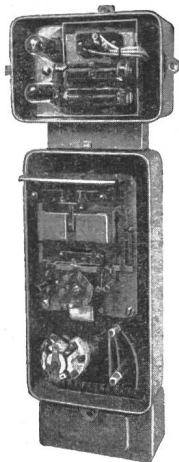
Fig. 1 Differential-Relais mit aufgebautelem Rückführgerät für Rheo-Flex-Regulierungen
