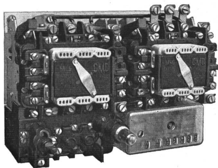
Fig. 1 Stern-Dreieck-Schutz 40 A
