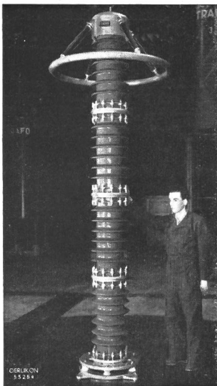
Fig. 1 Überspannungsableiter in neuer Bauart mit reduzierter Bauhöhe
