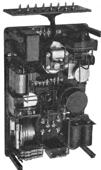
Fig. 3 Spannungs-Programmgler Innenansicht
