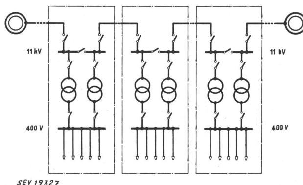
Fig. 17 Schalttechnischer Aufbau der englischen Transformatorstationen
