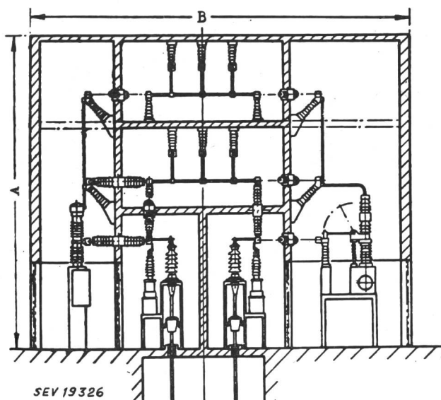
Fig. 16 Innenraumanlage für 66 bzw. 132 kV
