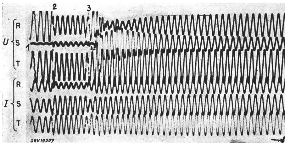
Fig. 7 Oszillogramm vom Beginn der Störung am 18. Juni 1951 Aufgenommen in Gösgen auf der Leitung Mettlen 2 (Lukmanierstrecke, A in Fig. 6)
