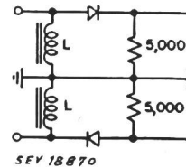
Fig. 18 Schaltung zur Erzeugung einer «geknickten» Sinus-Spannungskurve
