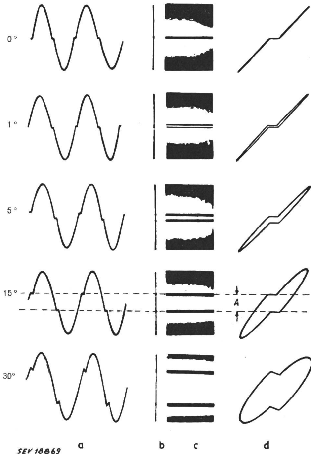
Fig. 19 Oszillogramme zur Phasenmessung mit einer «geknickten» sinusförmigen Wechselspannung Erklärungen siehe im Text
