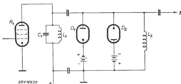
Fig. 7 Diodenbegrenzer
