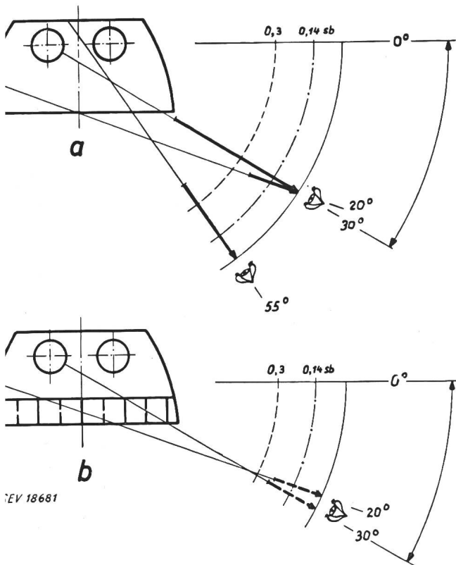
Fig. 8 Leuchtdichte in der Querebene bei der Leuchte Typ B a ohne Raster; b mit Raster; Maßstab 1 mm \cong 0,025 sb
