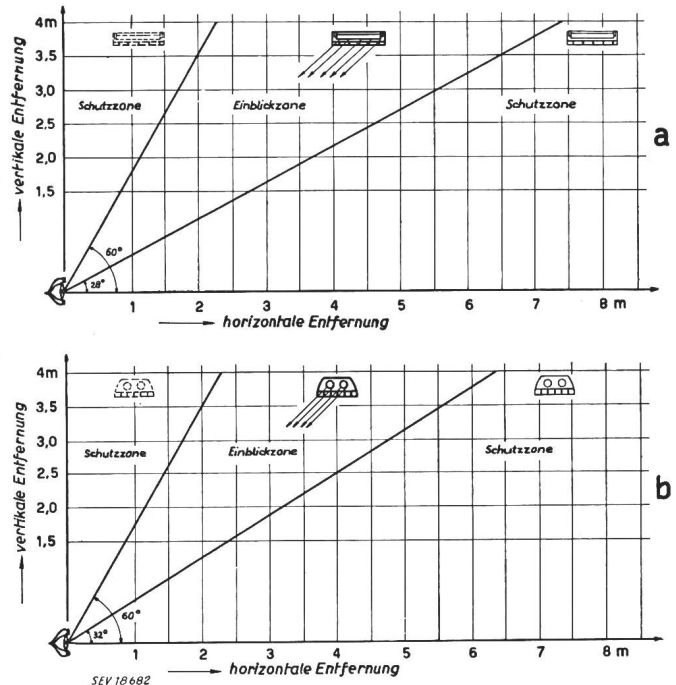
Fig. 9 Schutz- und Einblickzonen bei der Leuchte Typ B mit W-Raster a bei Längseinblick; b bei Quereinblick
