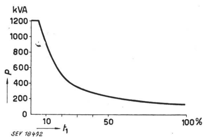
Fig. 6 Schaltleistung zweier Ignitrons in Gegentaktschaltung in Funktion der Einschaltdauer Grenzleistung = 1200 kVA, 380 V t_i Einschaltdauer (Integrationszeit = 8 s); P Leistung
