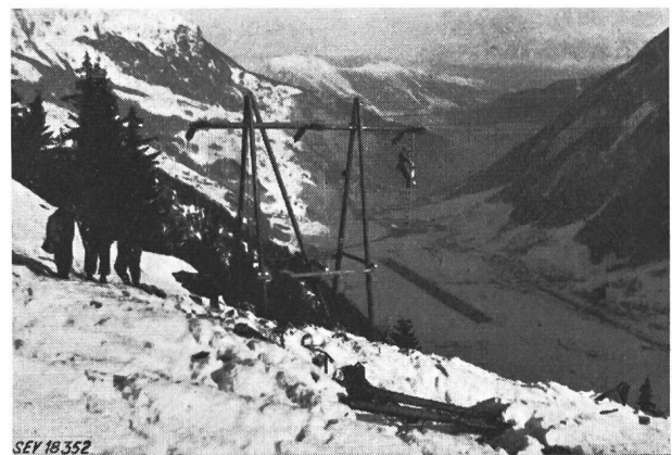
Fig. 11 Gotthardleitung Abspannmast aus Holz an der Unterbruchsstelle bei Mast Nr. 49 oberhalb Piotta
