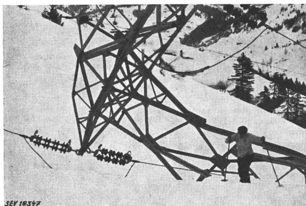
Fig. 6 Gotthardleitung Der zerstörte Mast Nr. 72 westlich Airola
