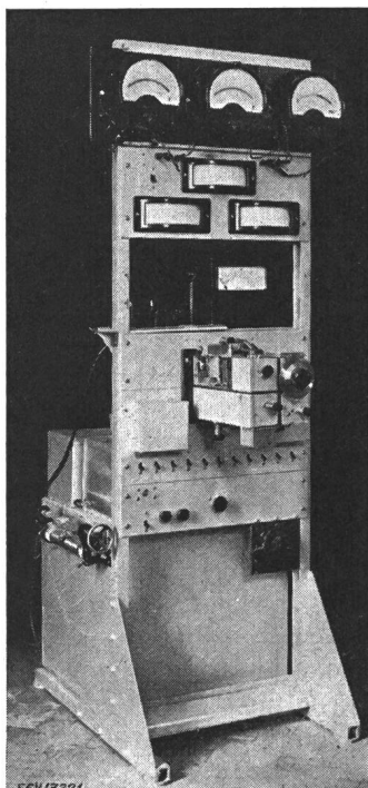
Fig. 5 Vorrichtung zur Messung der Eigenschaften von Überlagungsverstärkern mit Elektronenröhren bis etwa 200 MHz
