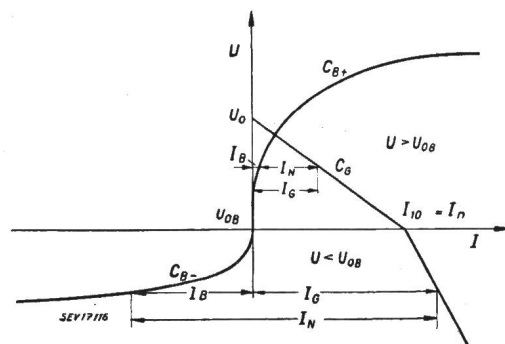
Fig. 15 Caractéristique statique d'une génératrice à shunt magnétique marchant en tampon avec une batterie d'accumulateurs (courbe de principe) C_G — caractéristique de la génératrice C_B + , C_B - — caractéristique de la batterie
