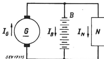
Fig. 14 Installation téléphonique avec marche en tampon (schéma de principe)
