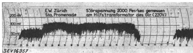
Fig. 2 Störspannungsdiagramm
