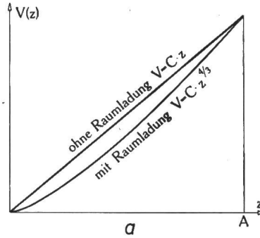
Fig. 9 Potentialverlauf und Elektronenbahnen in der ebenen Diode
