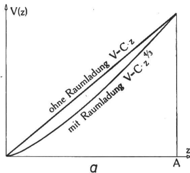
Fig. 9 Potentialverlauf und Elektronenbahnen in der ebenen Diode a Potential V_z in Funktion der Koordinate z b Elektronenbahnen mit und ohne Raumladung
