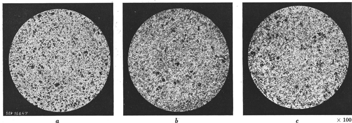
Fig. 10 Mikrogefüge des geglühten Rotorstahles mit Ni, V a; b; c wie bei Fig. 3
