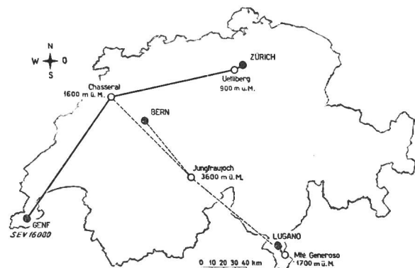
Fig. 1 Richtstrahl-Mehrkanalverbindung in der Schweiz
