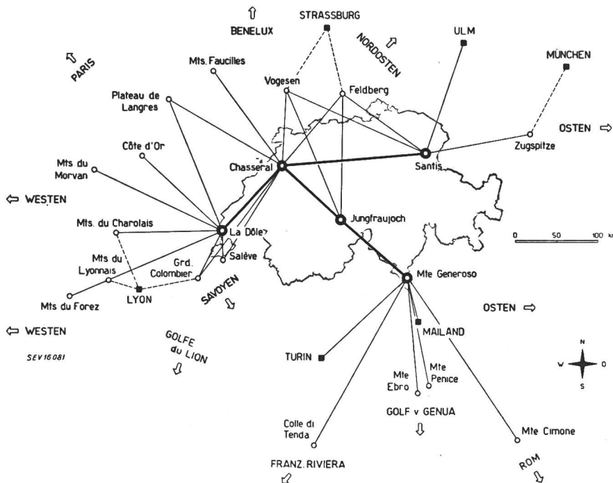
Fig. 2 Die internationalen Verbindungsmöglichkeiten des schweizerischen Mehrkanal-Richtstrahlnetzes
