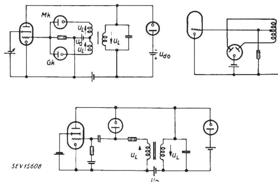
Fig. 8 Schaltungstechnische Ausführungen des Modells nach Fig. 6
