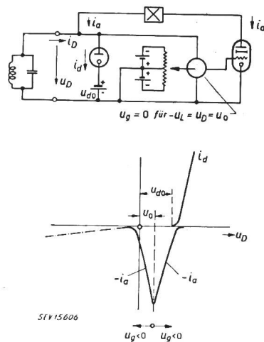
Fig. 6 Modell für automatische Umschaltung von Mit- auf Gegenkopplung und Kennlinie Die Gitterspannung wird mittels des Voltmeterzeigers abgegriffen
