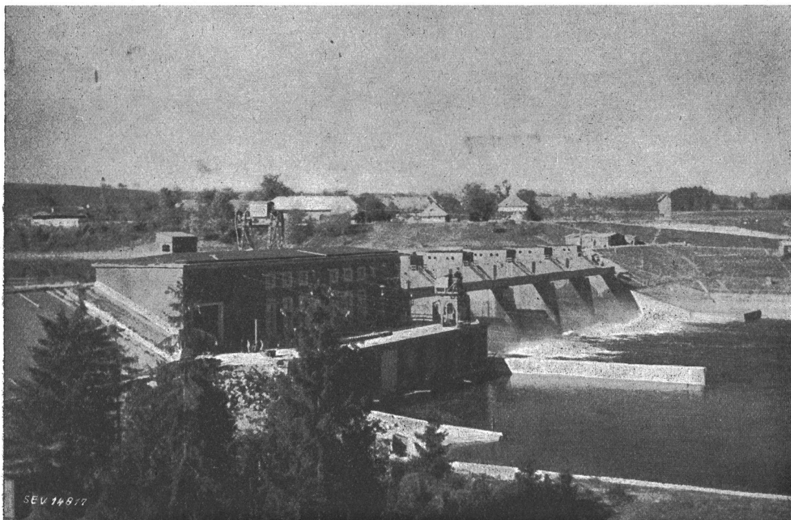
Fig. 1 Das Wasserkraftwerk Staning Ansicht von der Unterwasserseite
