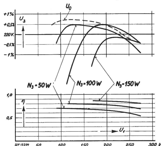
Fig. 4 Elektrische Daten des Stabilisators MST2
