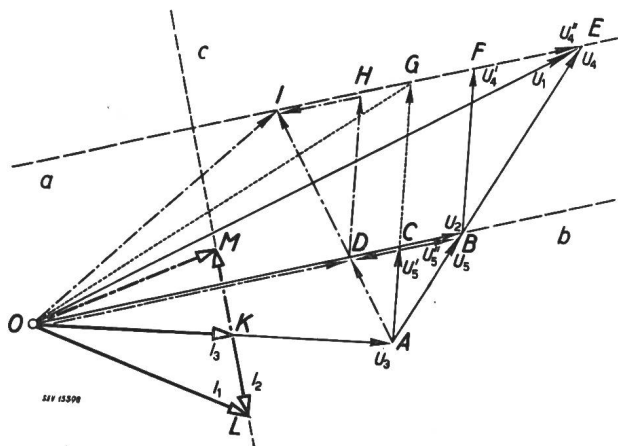
Fig. 3 Vektordiagramm der Teilspannungen eines magnetischen Stabilisators punktuelle Vektoren: Resonanzfall strichpunktuelle Vektoren: Netzspannung zu tief vollausgezogene Vektoren: Netzspannung zu hoch a geometrischer Ort der Spitze von U_1 ; b konstante Richtung von U_2 ; c geometrischer Ort von I_2
