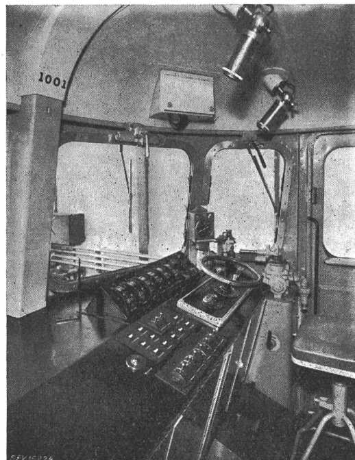
Fig. 3 Der Führerstand
