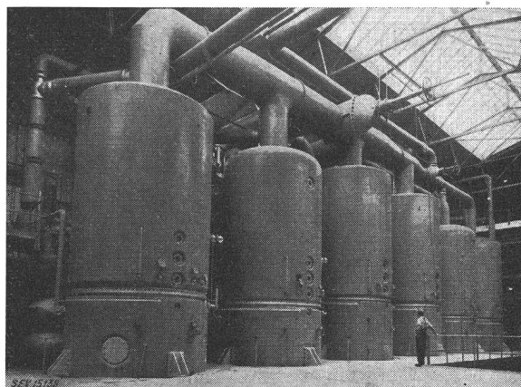
Fig. 5 Eindampfanlage
