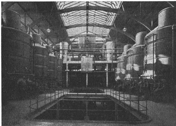
Fig. 7 Kochstation
