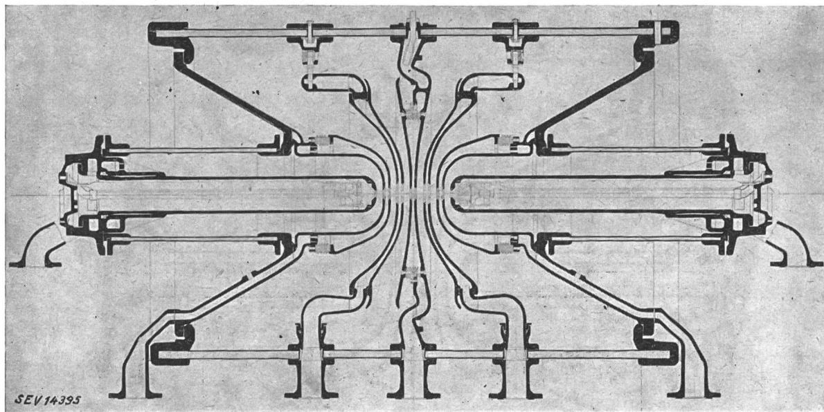
Fig. 5a Schnitt durch ein Marx-Ventil mit 6 Teilstrecken
