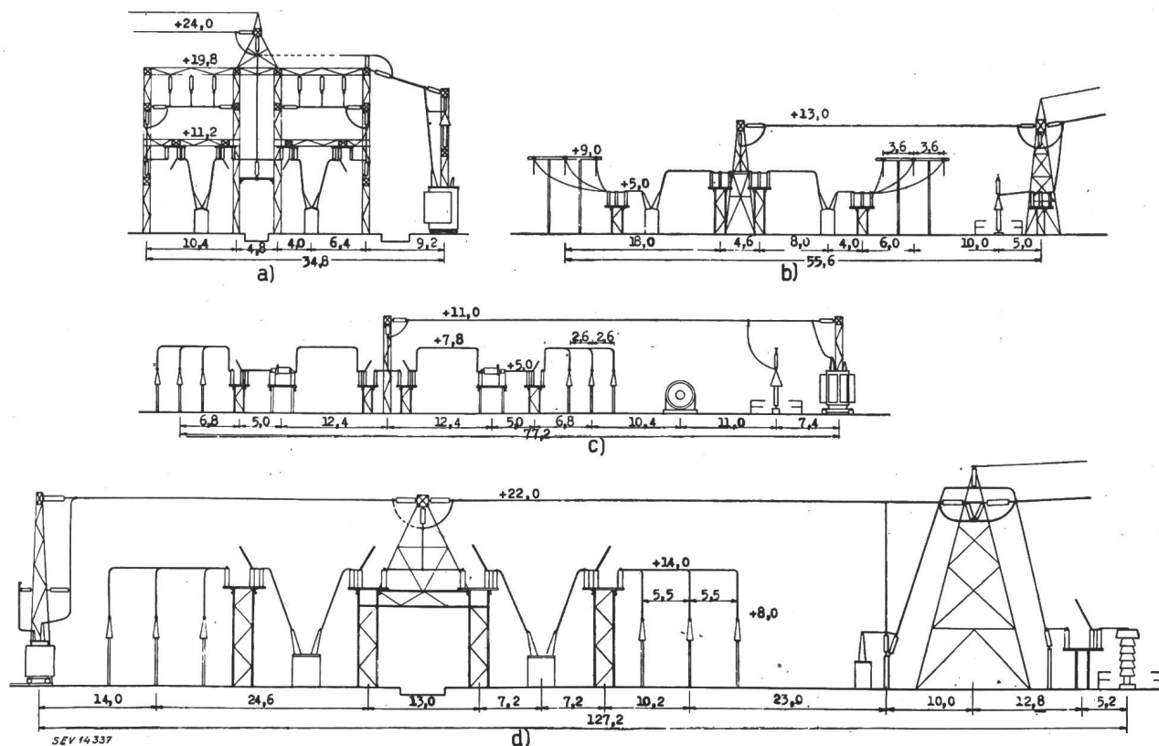
Fig. 2 Amerikanische Freiluftanlagen
