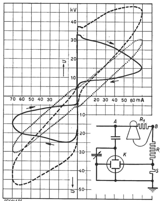
Fig. 1 Lichtbogen Pol-Erde über Isolator und nasse Stange Die Spannung am Isolator steigt bis 33 kV, der Lichtbogen zündet und die Lichtbogenspannung fällt bis zum Nulldurchgang. In der andern Phase der Wechselspannung ist der Verlauf symmetrisch.
