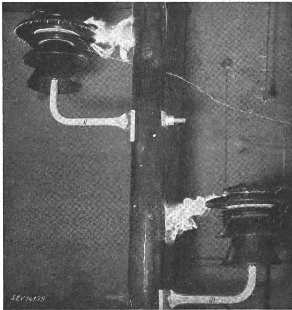
Fig. 9 Ueberschlag unter Regen 155 kV
