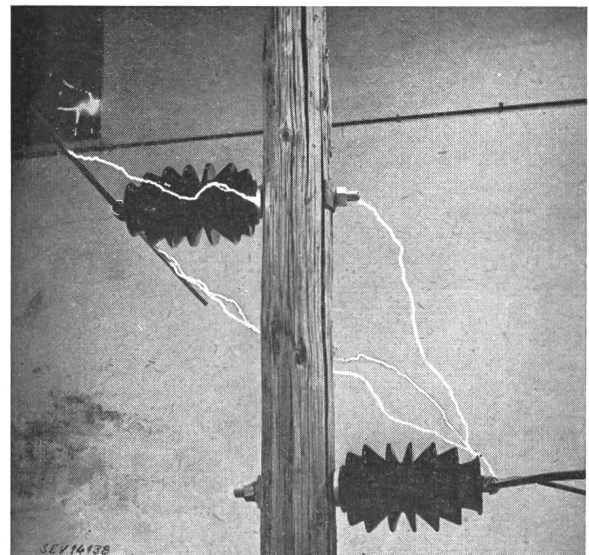
Fig. 8 50%-Stossüberschlag +605 kV (kleinster Wert)
