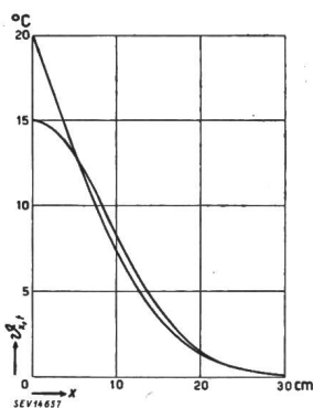
Fig. 7 zeigt die Ähnlichkeit der Temperaturfelder gleichen Wärmeinhaltes am Ende der Aufheizung und kurze Zeit nach Beginn der Abkühlung. Das Temperaturfeld des Abkühlungsvorganges hat nun gemäss (10) die Gleichung:
