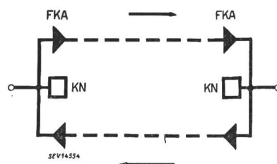
Vierdraht-Terminal
