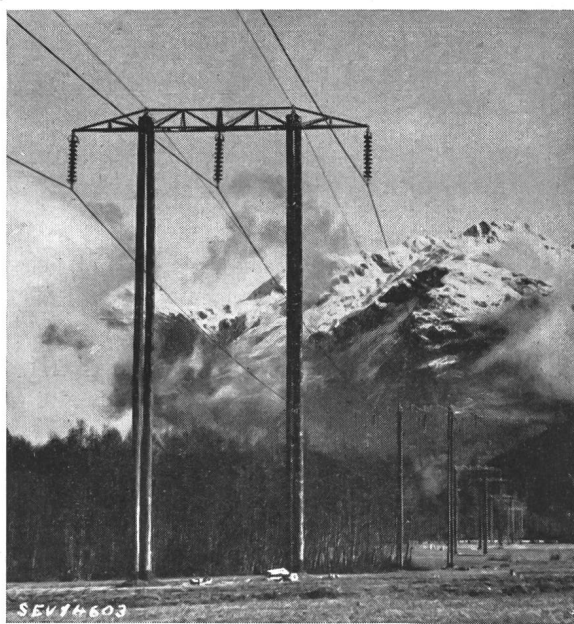
Fig. 6 Holztragmast mit 3 Reinaluminiumleitern von je 240 mm 2 und 2 Erdsellen von je 50 mm 2
