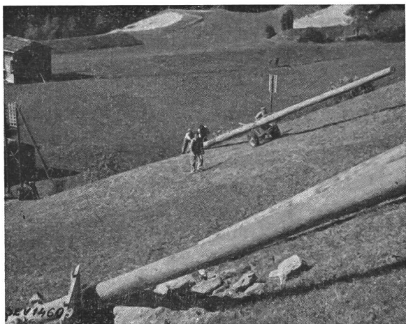
Fig. 12 Stangentransport mit Wagen und Winde
