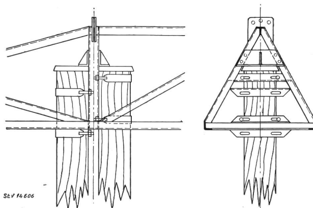
Fig. 9 Tragemast, Befestigung der Traverse an den Holzstangen Maßstab 1 : 25
