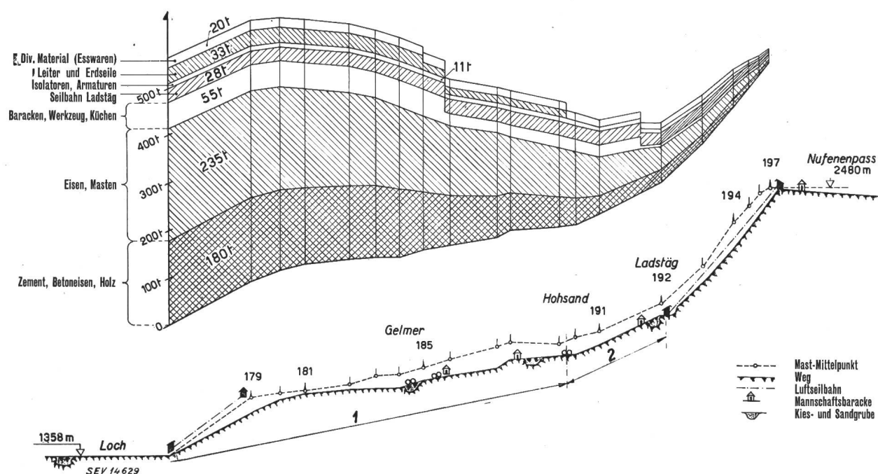
Fig. 28 Materialtransportgewichte der Gebirgsstrecke (über Transportweg aufgetragen) 1 mit Traktor befahrbare Strecke; 2 Maulesel-Transport
