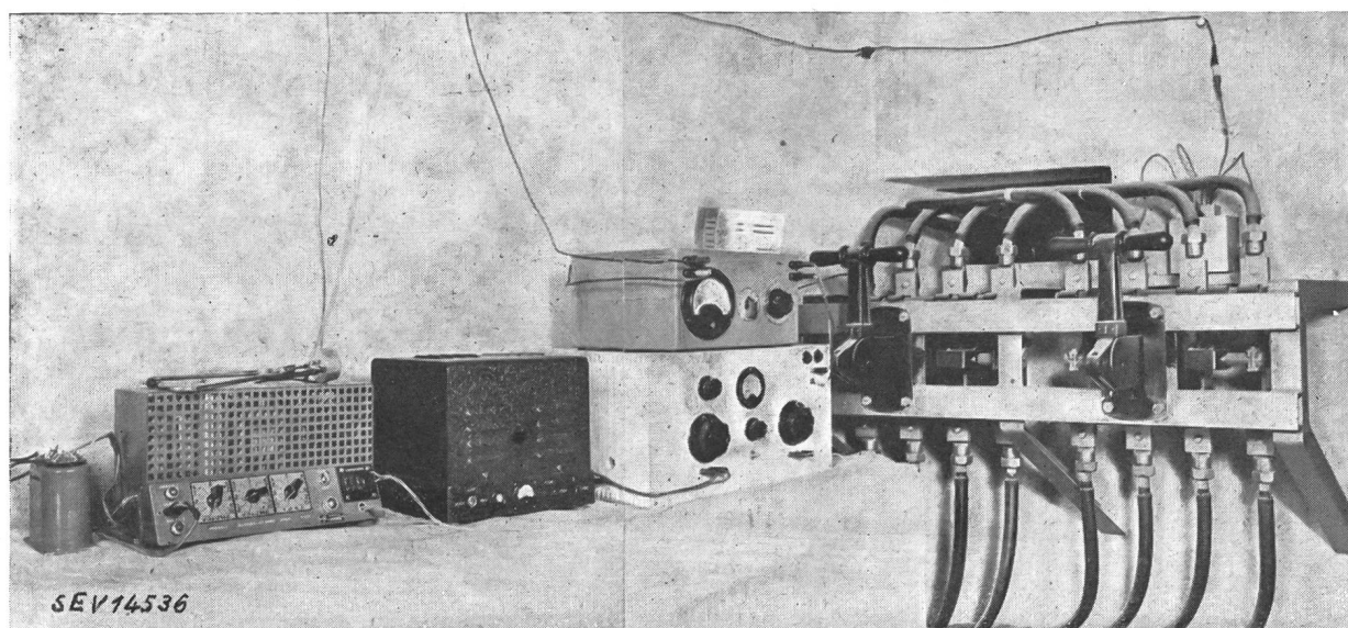
Fig. 1 Netzrundsprich-Versuchsanlage (Airolo)
