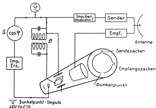
Fig. 6 Methode der Distanzmessung durch Kreisablenkung und Dunkelpunkt (Erläuterungen im Text)
