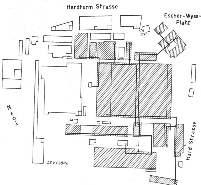
Fig. 11. Lageplan nach der Vereinheitlichung des Heizsystems Die schraffierten Gebäude werden aus der neuen Wärmezentrale mit Grundwasser-Wärmepumpe gespeist
