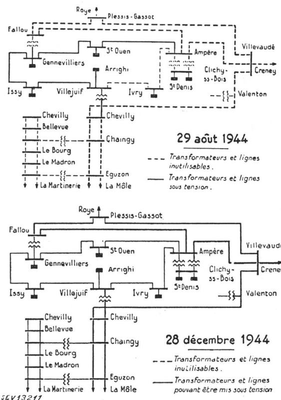
Fig. 1. Vereinfachtes Schema der Leitungen und Transformatoren in der Pariser Region
