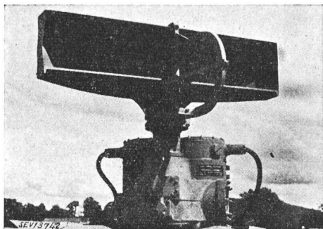
Fig. 2. Reflektor der 3-cm-Radar-Anlage
