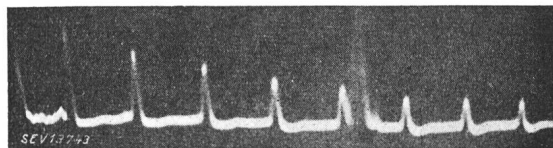
Fig. 3. Ausschnitt des Schirmbildes der Kontrollröhre Die Kurve zeigt 8 Distanzmarken und ein deutliches Echozeichen zwischen den Distanzmarken 5 und 6.
