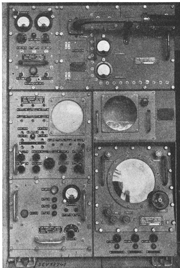
Fig. 1. Apparaterahmen der 3-cm-Radar-Anlage Linke Bildhälfte:
