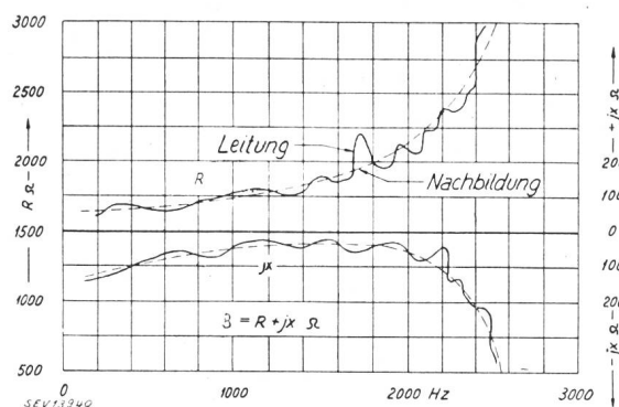
Fig. 3. Impedanzverlauf des Stammkreises einer Pupinleitung von 1 mm Aderdurchmesser Pupinisierung H-177-107.
