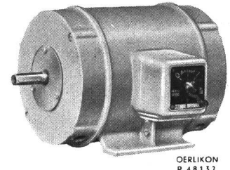
Fig. 6. Kleinmotor mit angebautes Schalter
