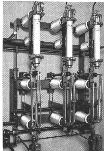
Fig. 2. Sectionneur auto-pneumatique de charge 20 kV, 150 et 400 A, combiné avec un coupe-circuit tripolaire
