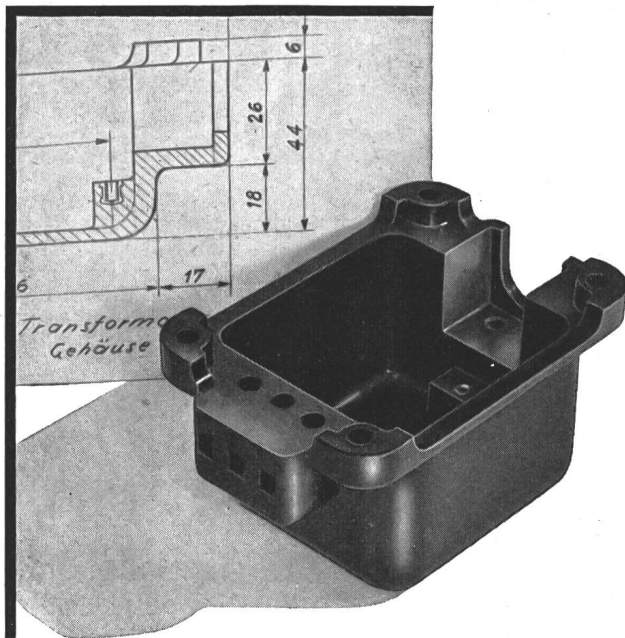
Fig. 1. Transformator-Gehäuse aus Kunstharz-Preßstoff
