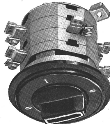
Fig. 3. Interrupteur «Multielle» pour commande de radiateurs ou de machines
