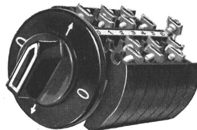
Fig. 4. Interrupteur «Combi» permettant toutes les combinaisons de schémas
