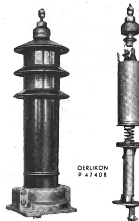
Fig. 4. Kondensator- Ueberspannungsableiter
