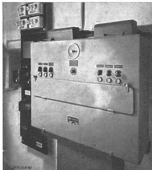
Fig. 1. Stufenschaltereinrichtung
