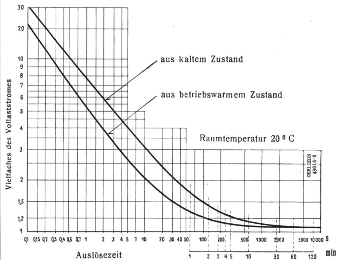
Fig. 2. Auslösecharakteristik der thermischen Ueberstromauslöser
