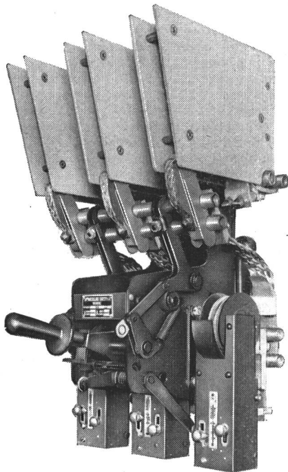
Fig. 1. Disjoncteur automatique tripolaire à rupture dans l'air, 100, 600 et 2000 A
