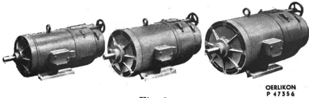
Fig. 7. Drehstrom-Nebenschluss-Kollektormotoren
