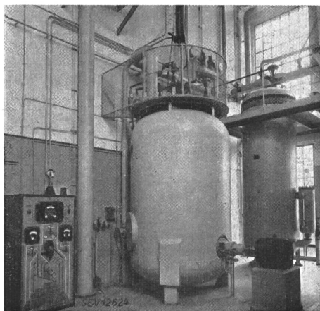
Fig. 1. Sulzer-Elektro-Heisswasserkessel 5000 kW, 6 kV, 12 kg/cm 2 Betriebsdruck, in einem Fernnetzwerk
