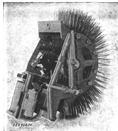
Fig. 1. Chercheur à 30 positions un nouvel élément des centraux téléphoniques automatiques Hasler
