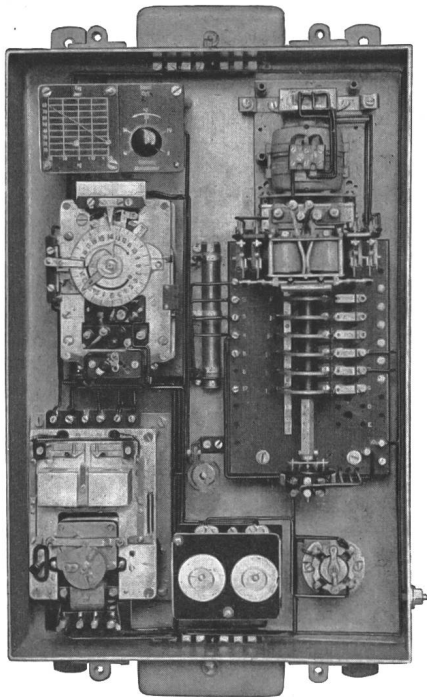
Fig. 1. Equitherm-Regulierung
