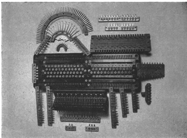
Fig. 1. Presstelle aus Suconit
