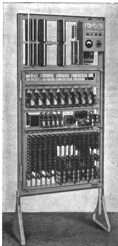
Fig. 1. Ansicht der offenen Hauszentrale für 20 Teilnehmer und 3 Amtsleitungen
