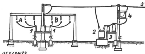
Fig. 2. Halbhohe Mittelmastbauweise
