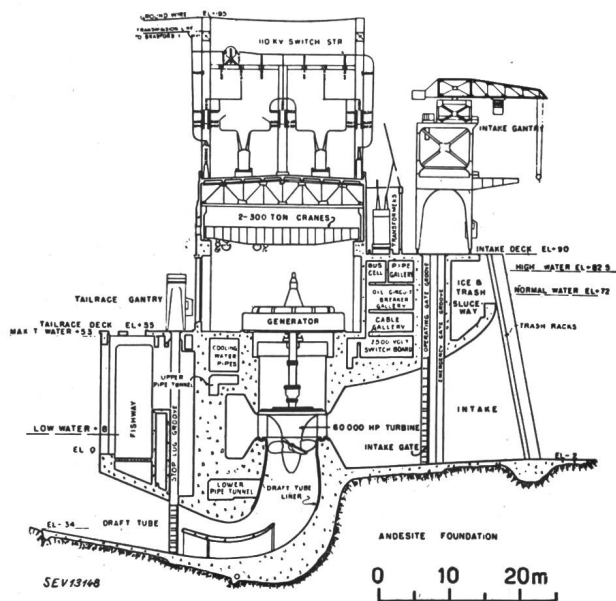
Fig. 11. Bonneville Maschinenhausquerschnitt
