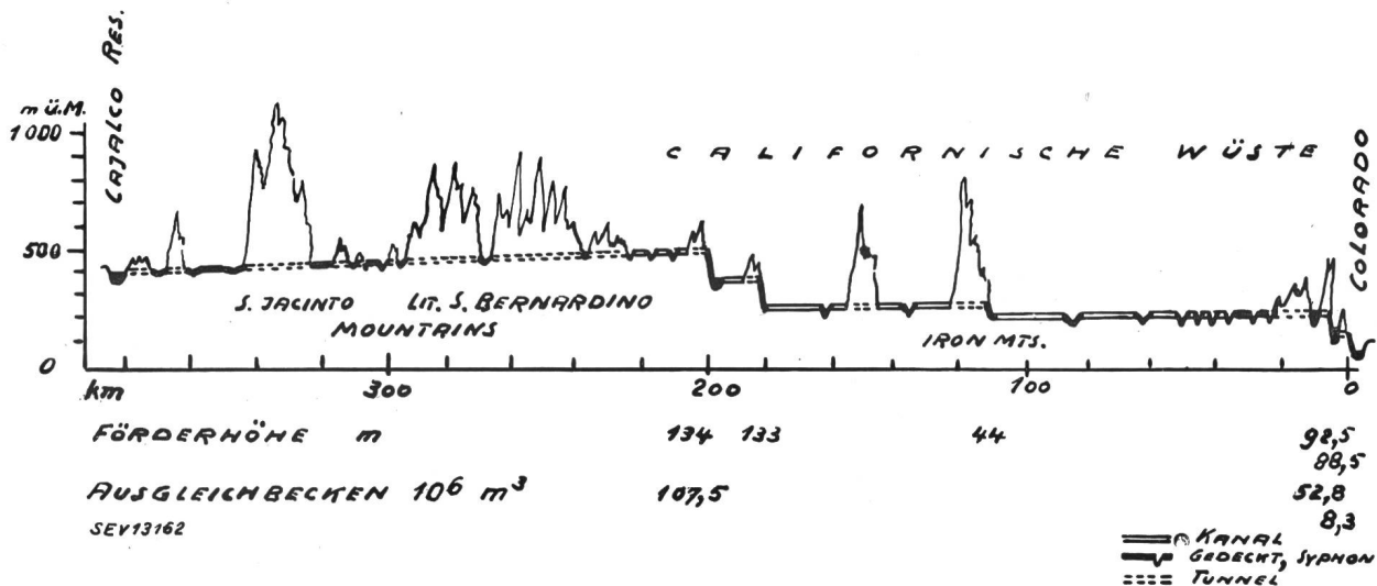
Fig. 25. Längensprofil des Metropolitan Aqueductes
