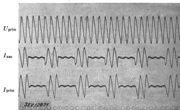
Avec condensateur série
