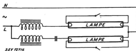
Fig. 2. Schema der Paar-Schaltung zur Verminderung der Welligkeit des Lichtes
