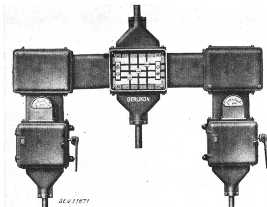
Fig. 1. Verteilbatterie mit 2 Schaltkasten mit Sicherungen 25 A, 500 V Deckel am mittleren der Verteilkasten weggenommen.
