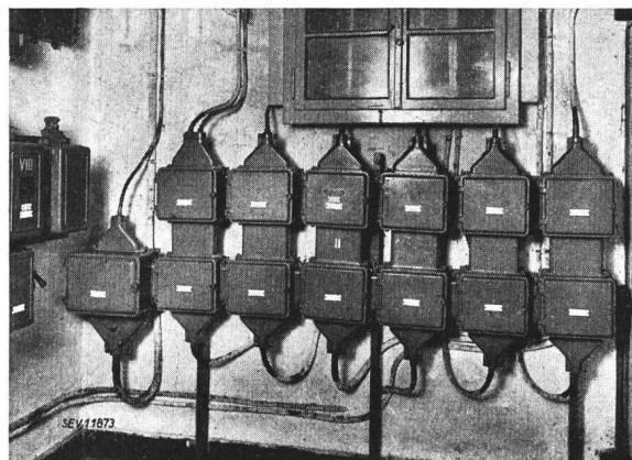
Fig. 3. Sicherungskastenbatterie 500 V, 150 A
