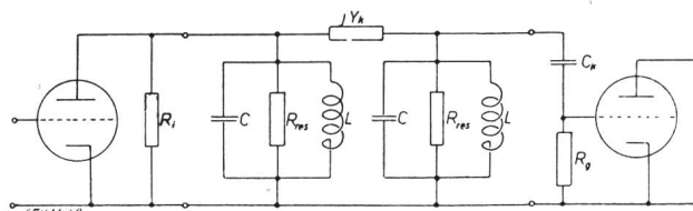
Fig. 1. Schema eines zweikreisigen Bandfilters
