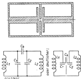
Fig. 3. Kapazitiv gekoppeltes Bandfilter Oben: Schnitt. Unten: Ersatzschema.
