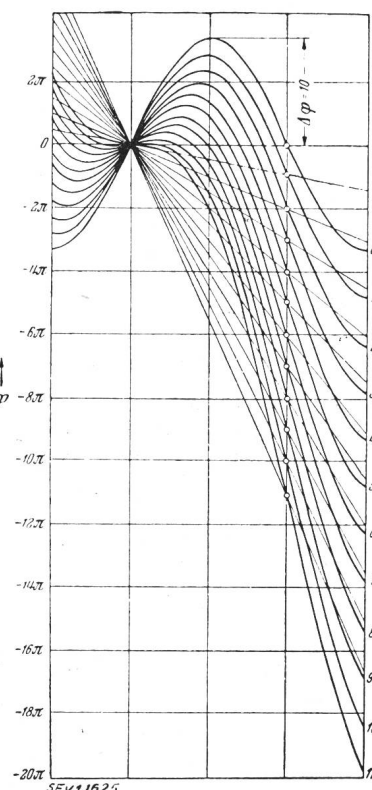
Fig. 5. Phasenwinkelverlauf bei verschieden hoher Überlagerungsfrequenz
