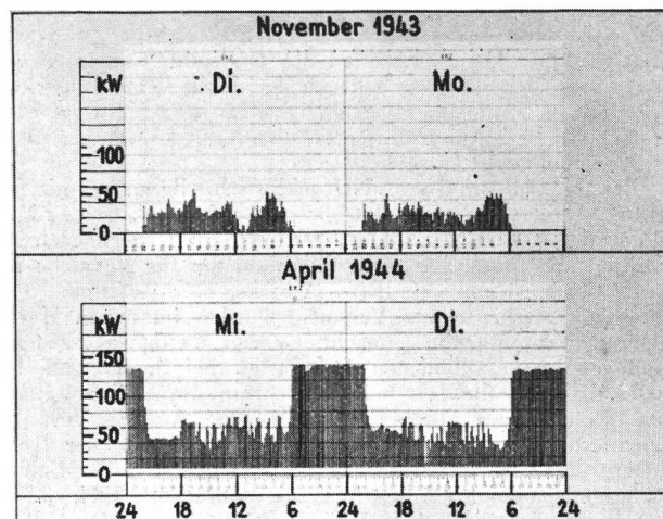
Fig. 2. Textilbetrieb Bezug und Rücklieferung von Energie.
