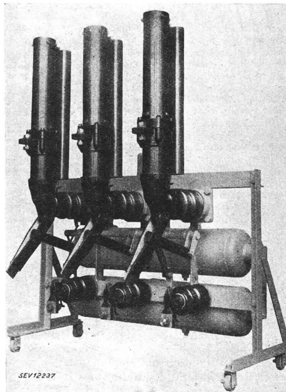
Fig. 2. Druckluftschnellschalter mit Fahrgestell und Zusatzbehälter für Wiedereinschaltung Nennspannung 20 kV, Nennstrom 1000 A, 600 MVA Abschaltleistung.
