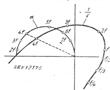
Fig. 7. a -Kurve, bei der der Verstärker schwingt
