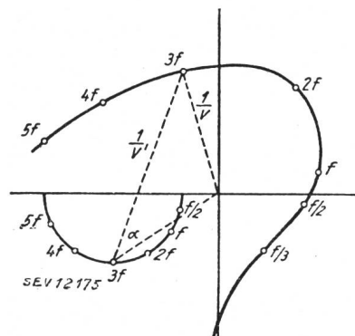
Fig. 6. Zeichnerische Bestimmung von \frac{1}{v'} aus \frac{1}{v} und a
