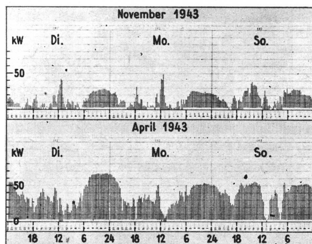
Fig. 3. Wiederverkäuferwerk Bezug und Rücklieferung von Energie.
