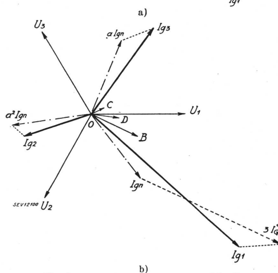
Fig. 3a Diagrammes des courants dans la ligne g a) pour réseau à neutre isolé. b) pour réseau avec bobine d'extinction.
