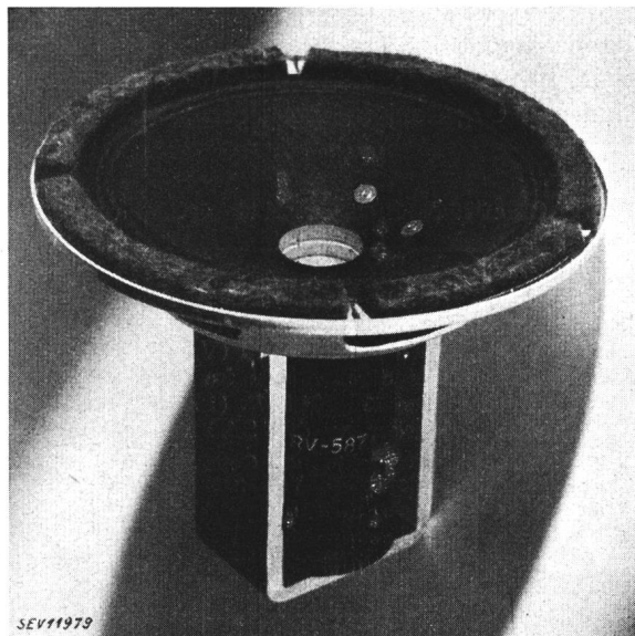
Fig. 1. Dynamischer Wandler
